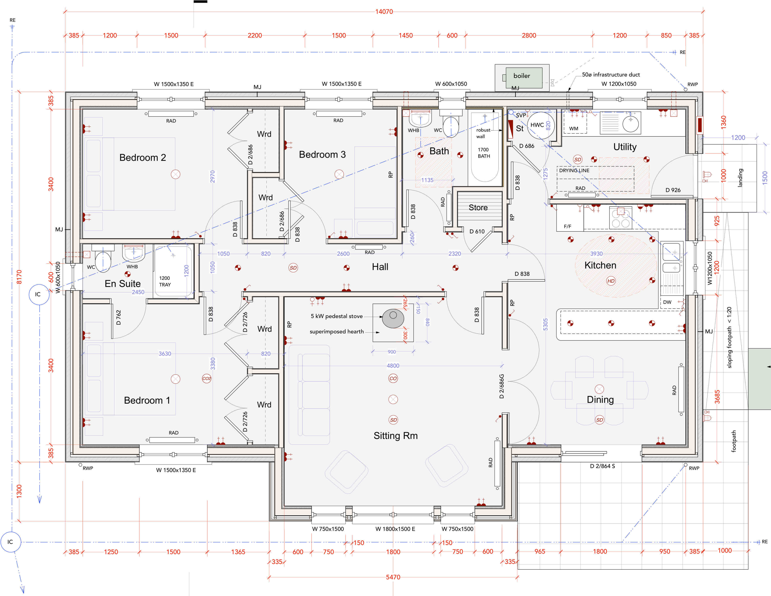
Floor Plan 105.0 m2 Scale: 1:50
